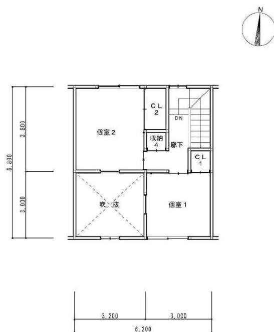
2階平面図 1 : 1 0 0
