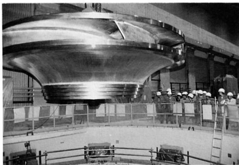
▲ゆっくりとランナが4号機にすえつけられる
