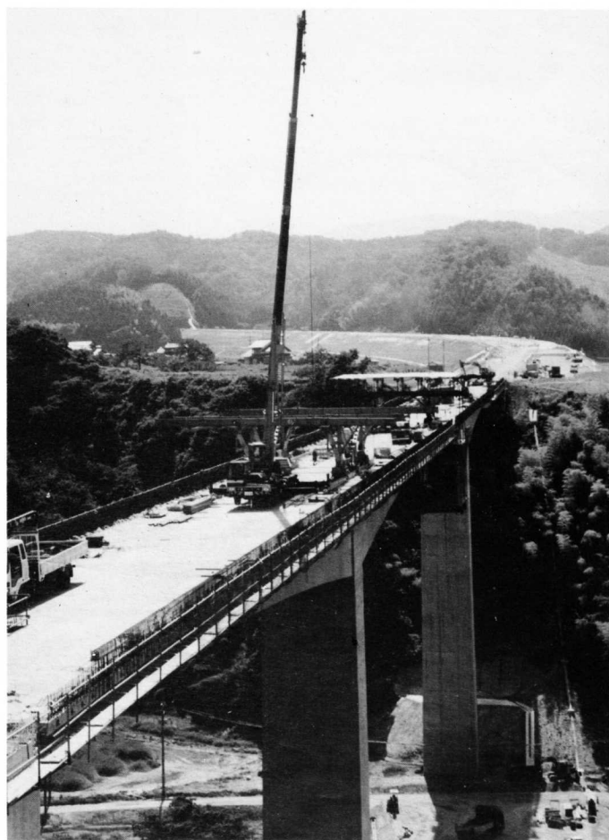
▲完成真近な船谷川橋から岡山方面にのびる横断面
